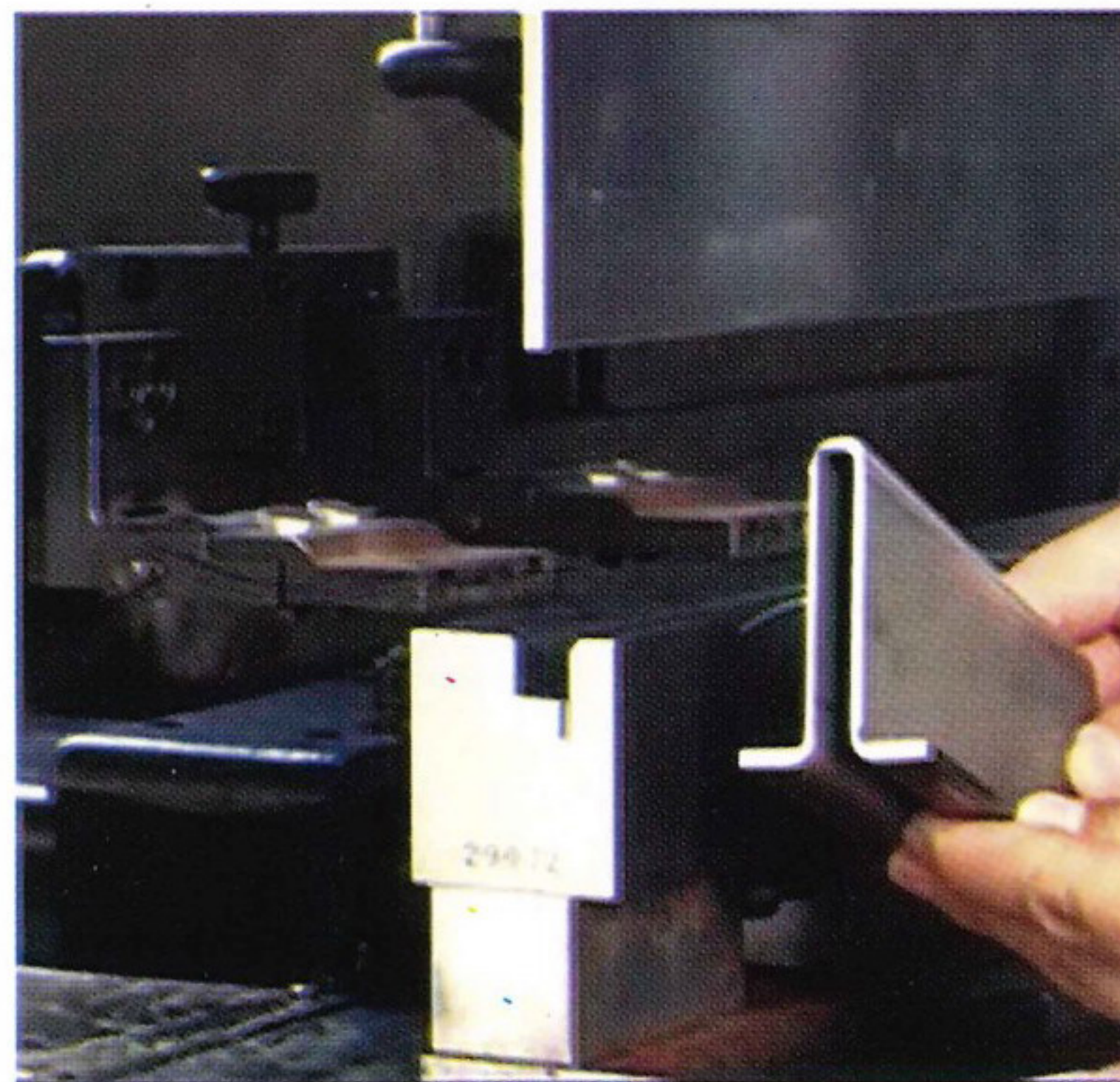
U channel die
