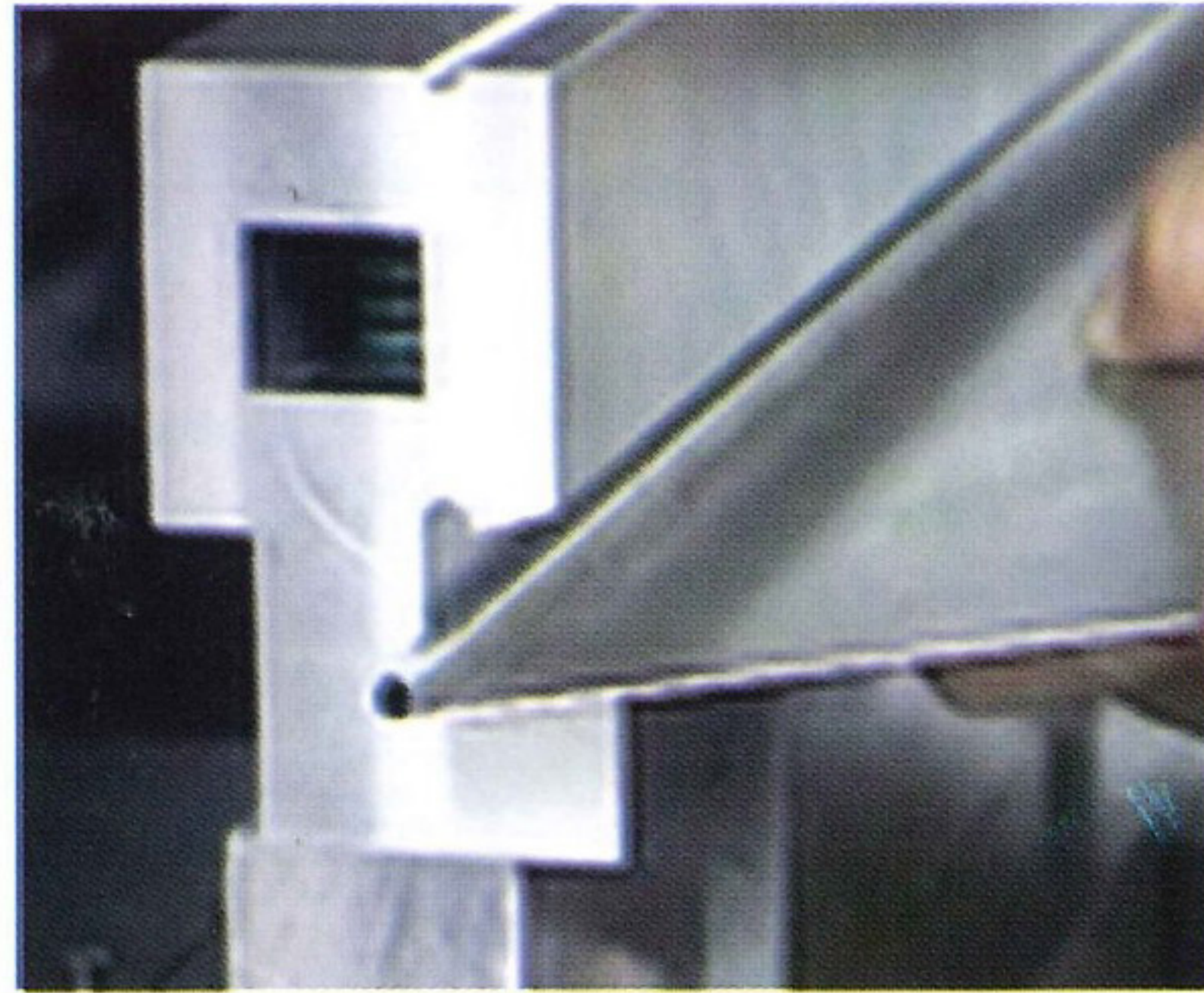
Curling Die
